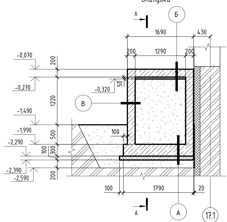
Б-Б Опалубка
