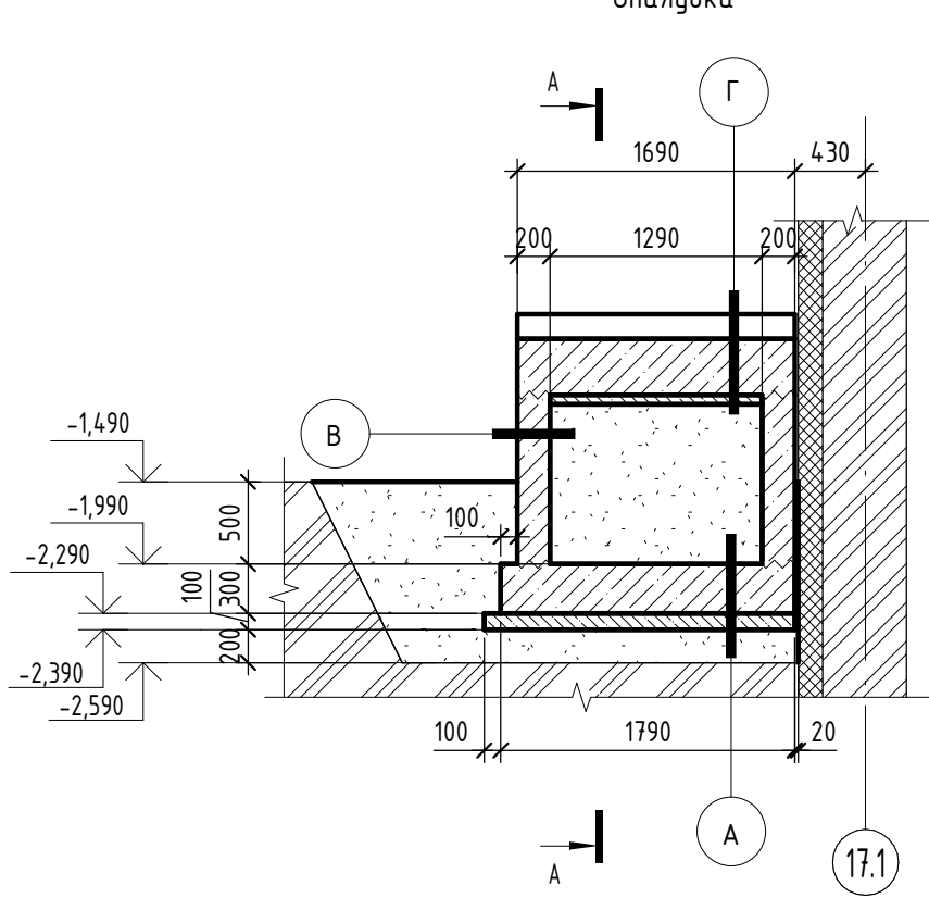
В-В Опалубка
